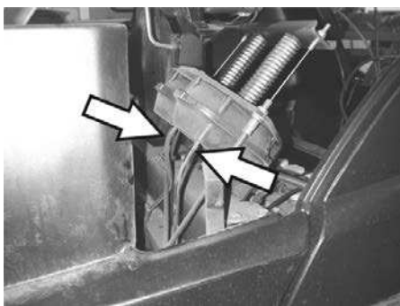
Slangetilslutning til undertryksdåsen af fejervalsens sænkning
