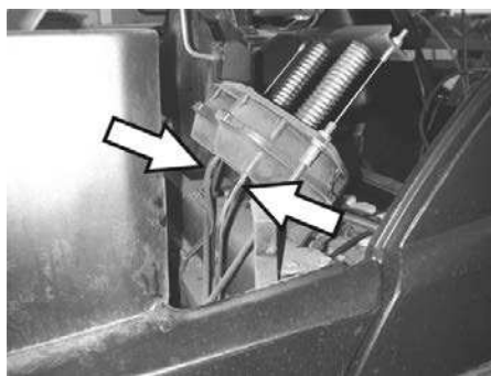
Priklučki gibke cevi do podtlačne doze spuščanja pometalnega valja
