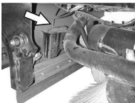
Элемент подключения шланга для мембранного механизма вакуумного регулятора опускания боковых щеток.
