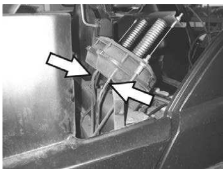
Przłącza węży do puszek podciśnieniowej mechanizmu opuszczania walca zmiatającego
