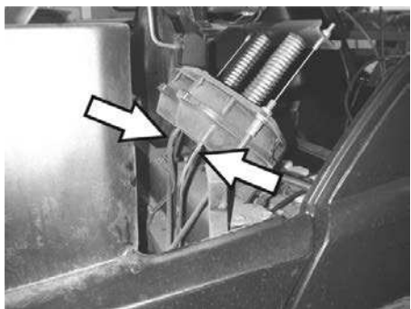
Συνδέσεις ελαστικών σωλήνων με το κιβώτιο χαμηλής πίεσης για το χαμάλωμα του κυλίνδρου σκουπίσματος
