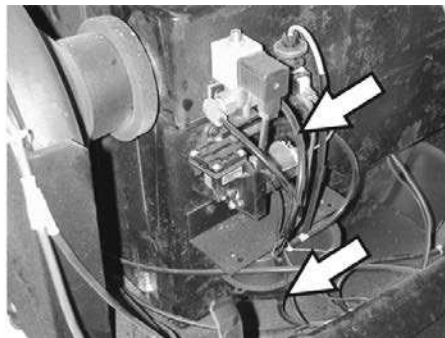
Slangetilslutningerne til undertryksdåsen og undertryksdåsen (lager)
