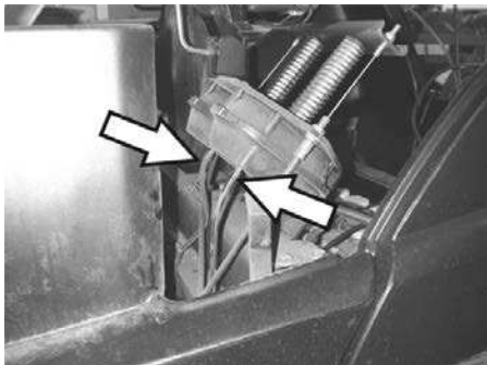
Lakaisutelan alaslaskun alipainerasian letkuliitäntä
