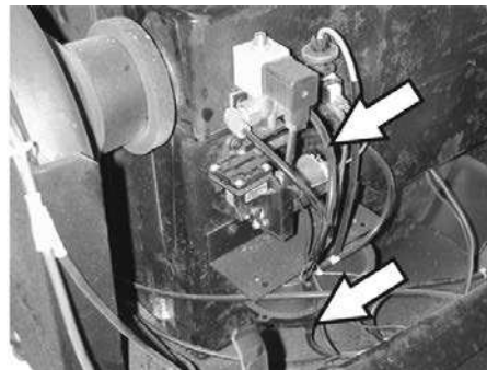
Priklučki gibke cevi do podtlačne črpalke in do podtlačne doze (zbiralnik)
