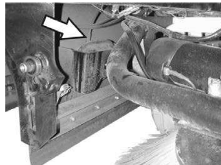
Schlauchanschluss zur Unterdruckdose der Seitenbesenabsenkung
