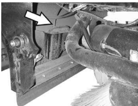
Sivuharjan alaslaskun alipainerasian letkuliitäntä
