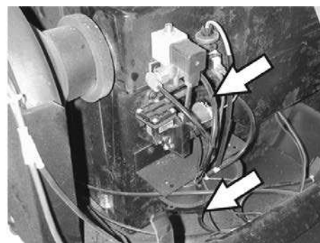
Tömlőcsatlakozás a vákuumszivattyúhoz és a vákuumszelencéhez (tároló)
