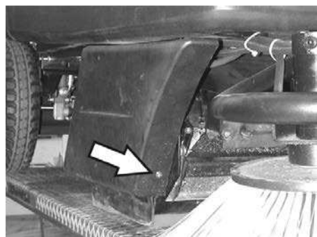
Tömlőcsatlakozás a seprőhenger leengedés vákuummérő szelencéjéhez
