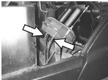
Hadicové přípojky k podtlakové nádobě pro snižování zemetacího válce
