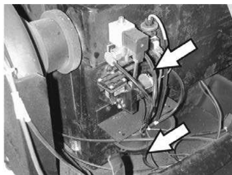
Підключення шлангів до вакуумного насоса та до мембранного механізму вакуумного регулятора (ресивер)
