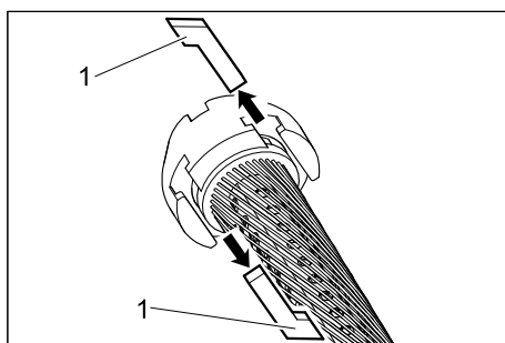
1 Γλωσσίδα
