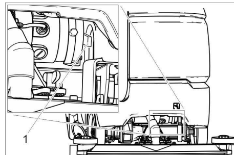
1 Uvoľňovacia páka
