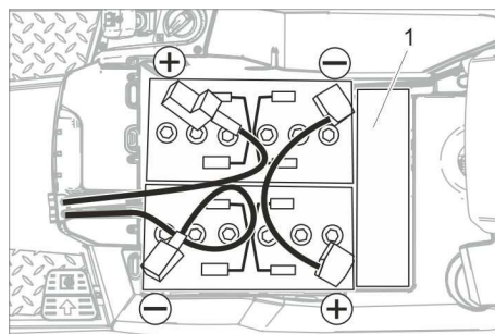
1 Разпорен елемент
