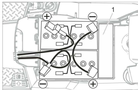
1 Distančnik
