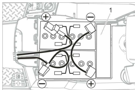
1 Distanční vzpěra
