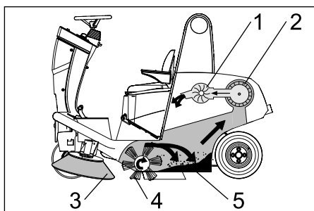
Rys. 1 Zamiatarka pracuje na zasadzie przerzucania.
